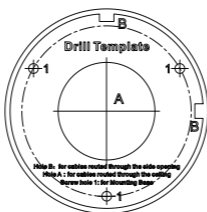
Рисунок 2-4 Шаблон крепления монтажной коробки
