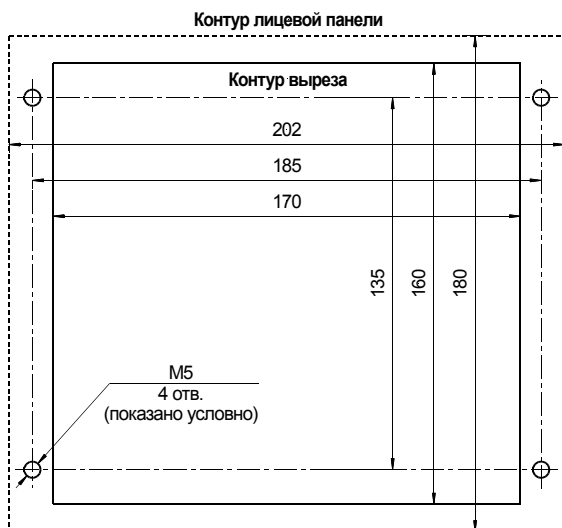
Рис. 1. Разметка под установку блока вызова.
