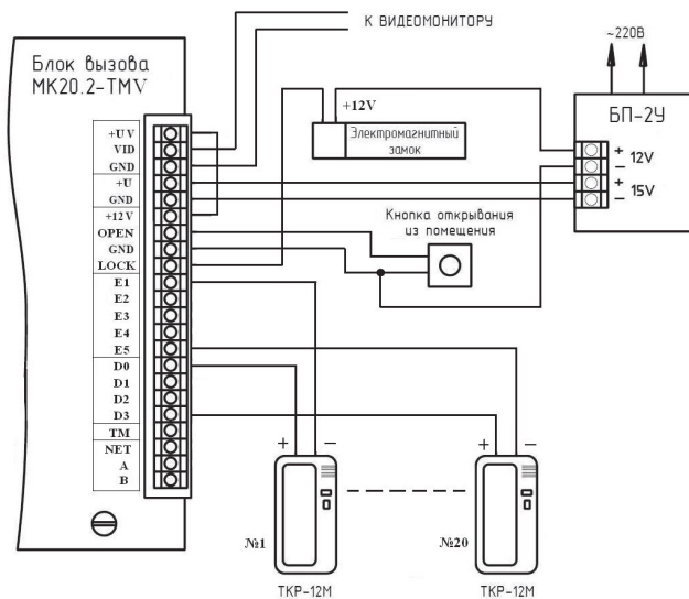
Рис. 2 Пример монтажа блока вызова МК20.2-TMV
