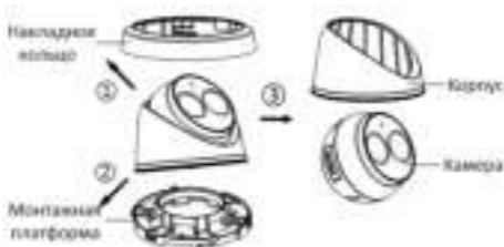
Рисунок 2-15 Демонтаж камеры
