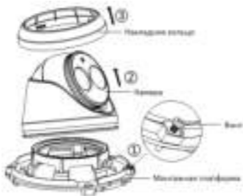
Рисунок 2-1 Демонтаж камеры
