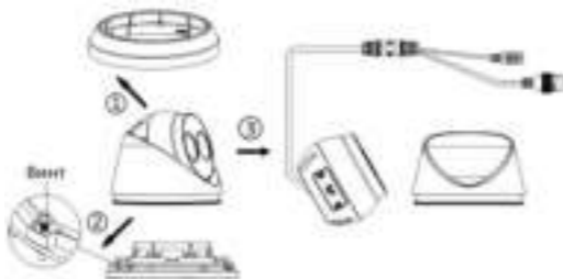
Рисунок 2-23 Демонтаж камеры
