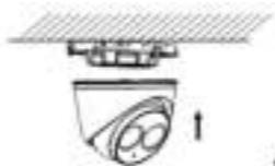
Рисунок 2-20 Установка камеры
