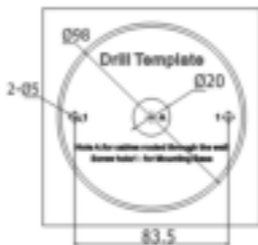
Рисунок 2-18 Шаблон крепления
