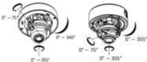
Рисунок 2-10 3-х осовая установка (Слева) Камера II типа (Справа) Камера III типа
