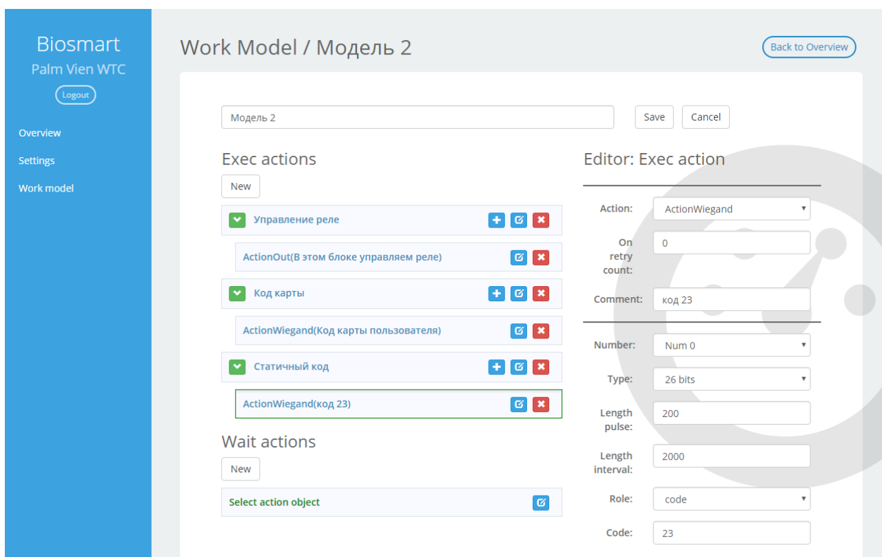
Рисунок 70. Создание сценария
