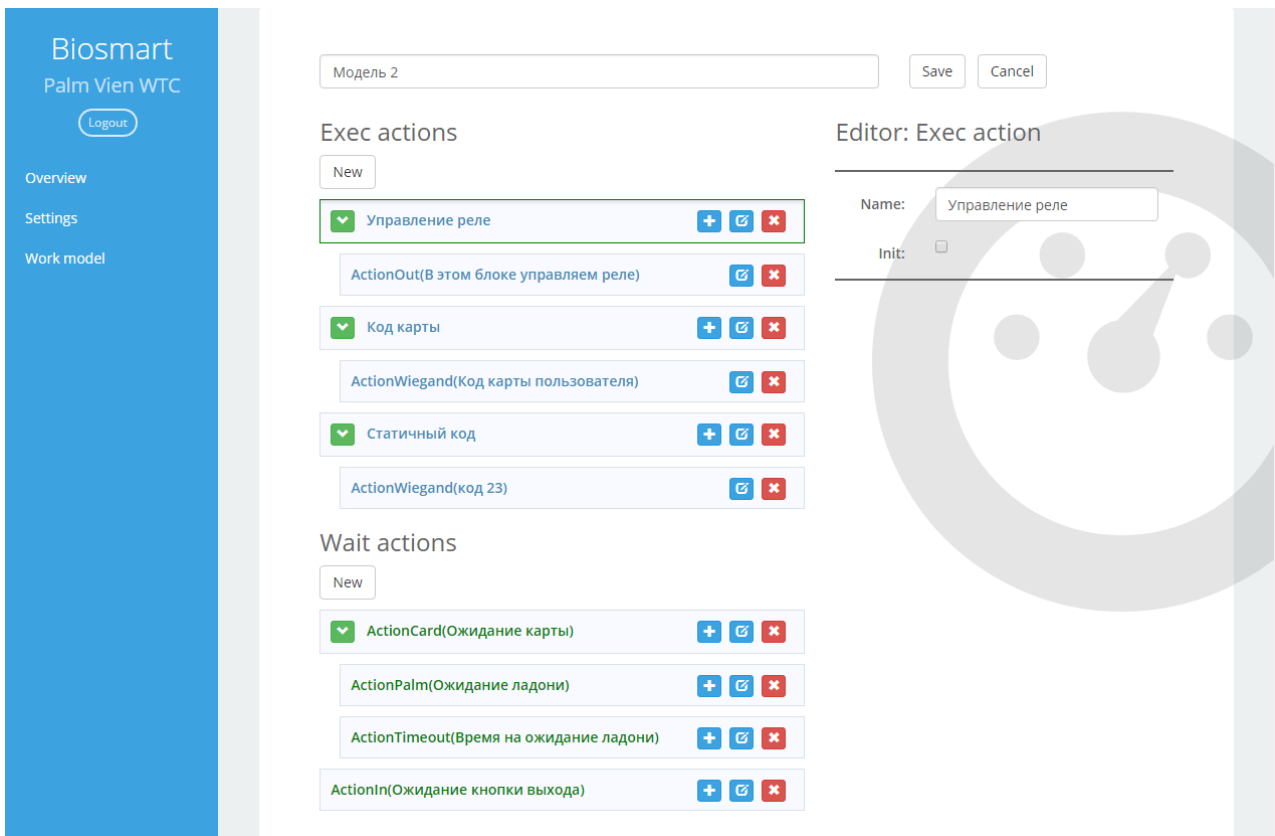
Рисунок 67. Готовый сценарий
