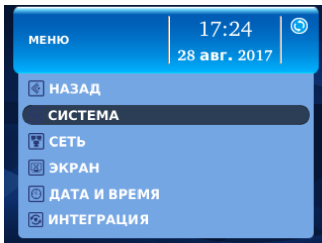
Рисунок 6. Система
