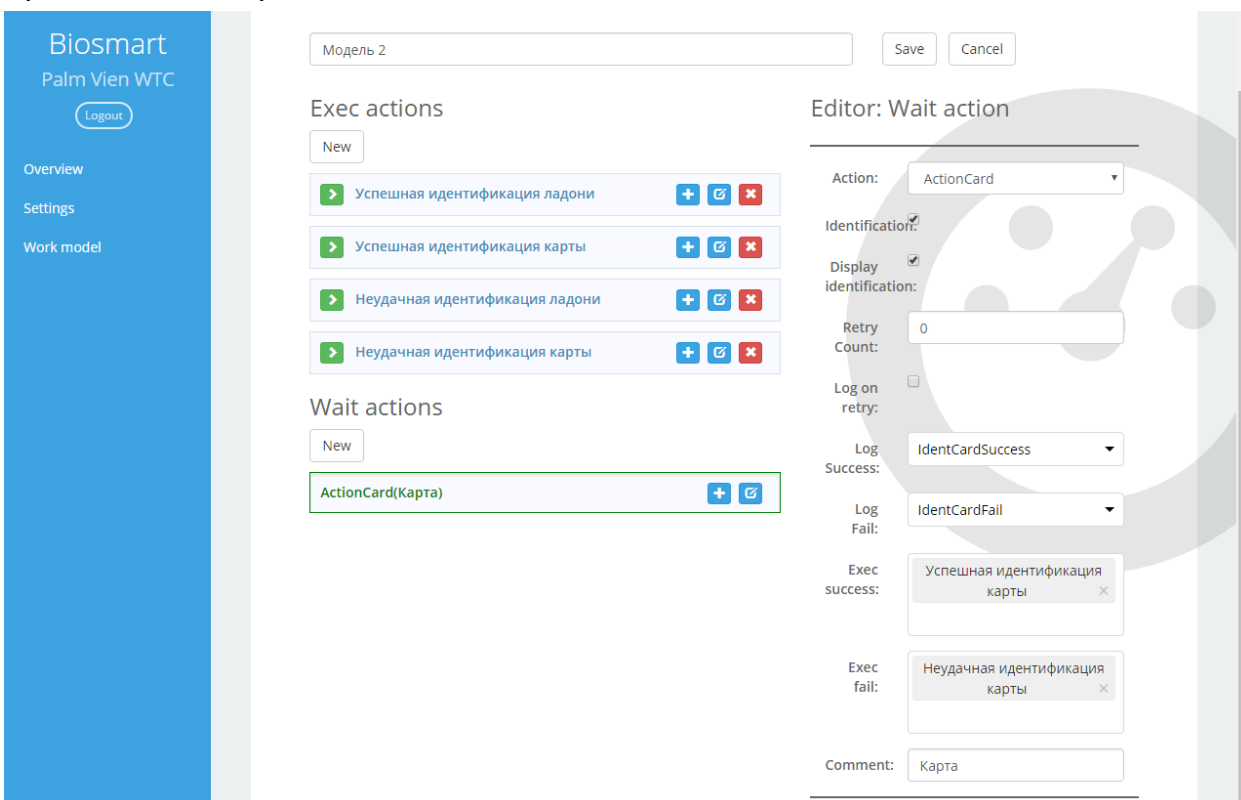
Рисунок 65. Создание сценария
