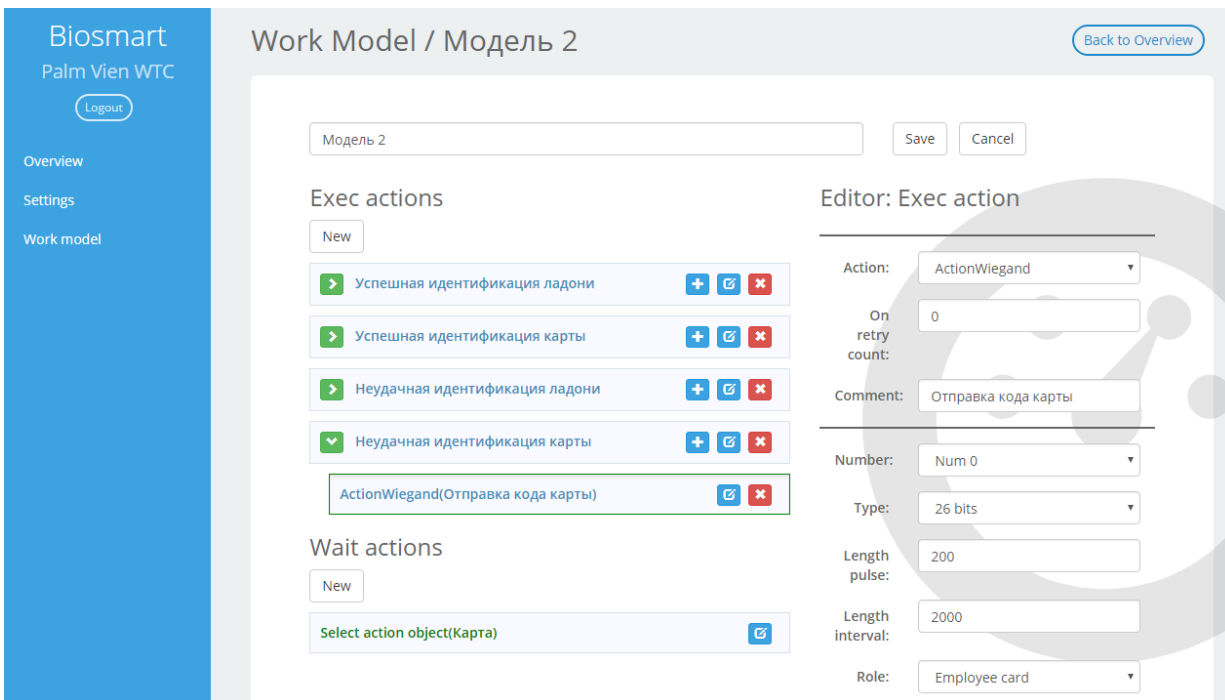
Рисунок 64. Создание сценария
