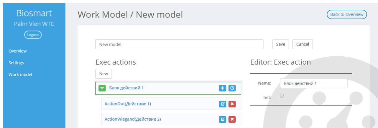
Рисунок 51. Блок действий
