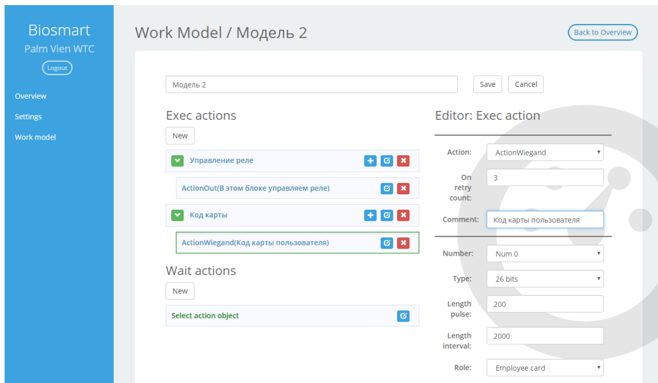
Рисунок 69. Создание сценария.
