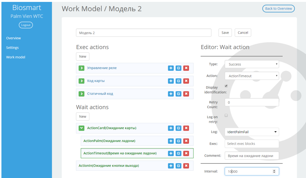
Рисунок 73. Создание сценария
