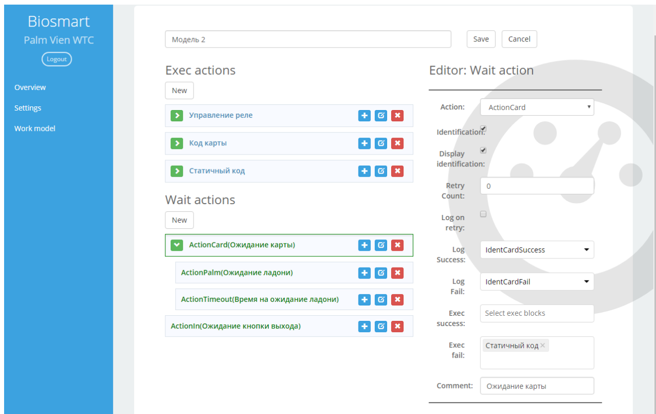
Рисунок 71. Создание сценария
