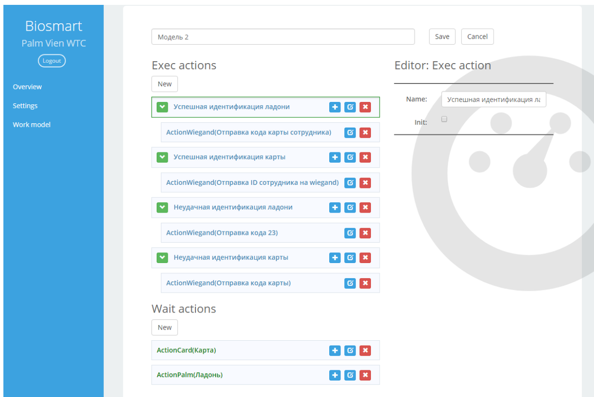
Рисунок 60. Готовый сценарий
