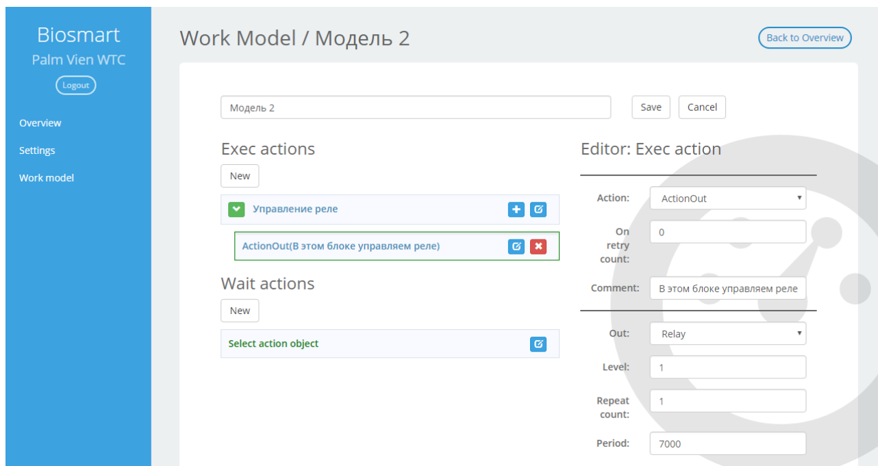
Рисунок 68. Создание сценария.
