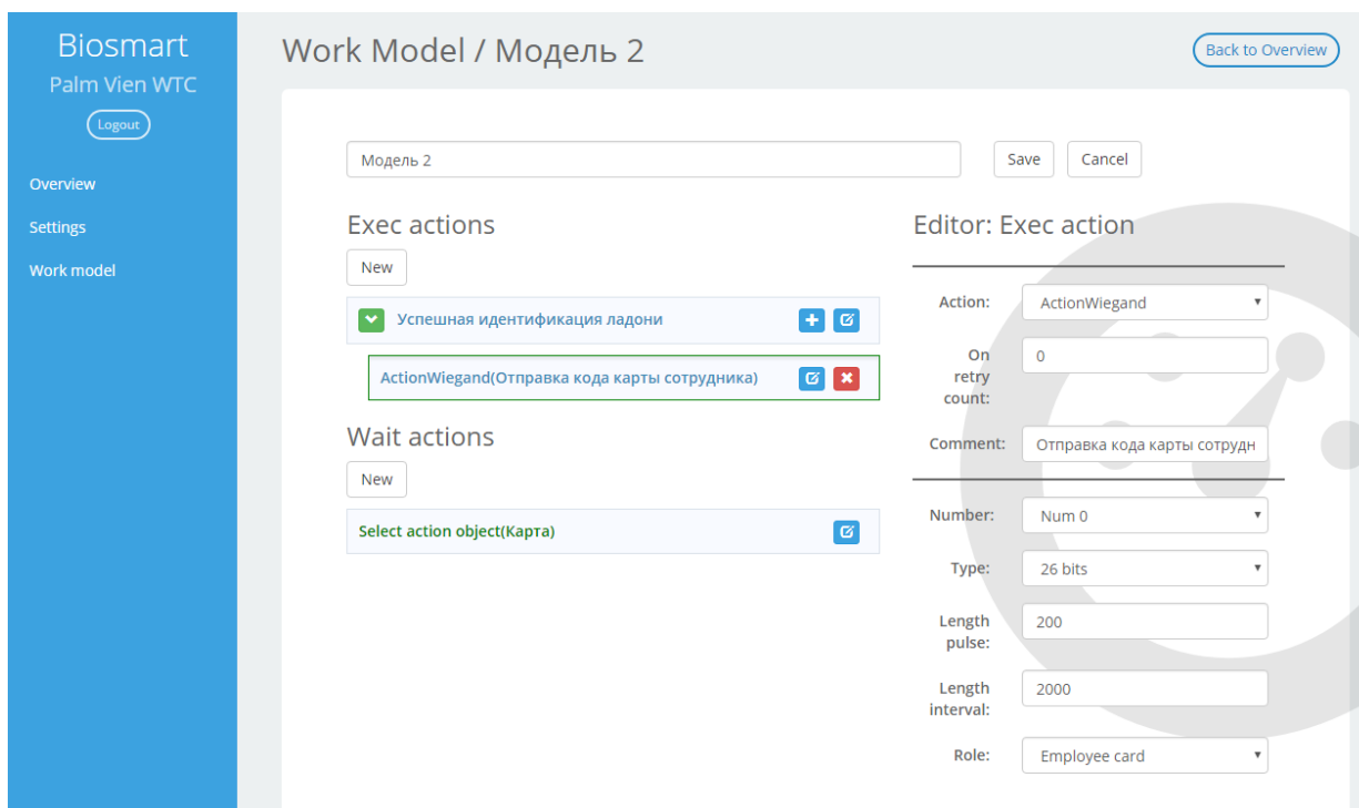
Рисунок 61. Создание сценария
