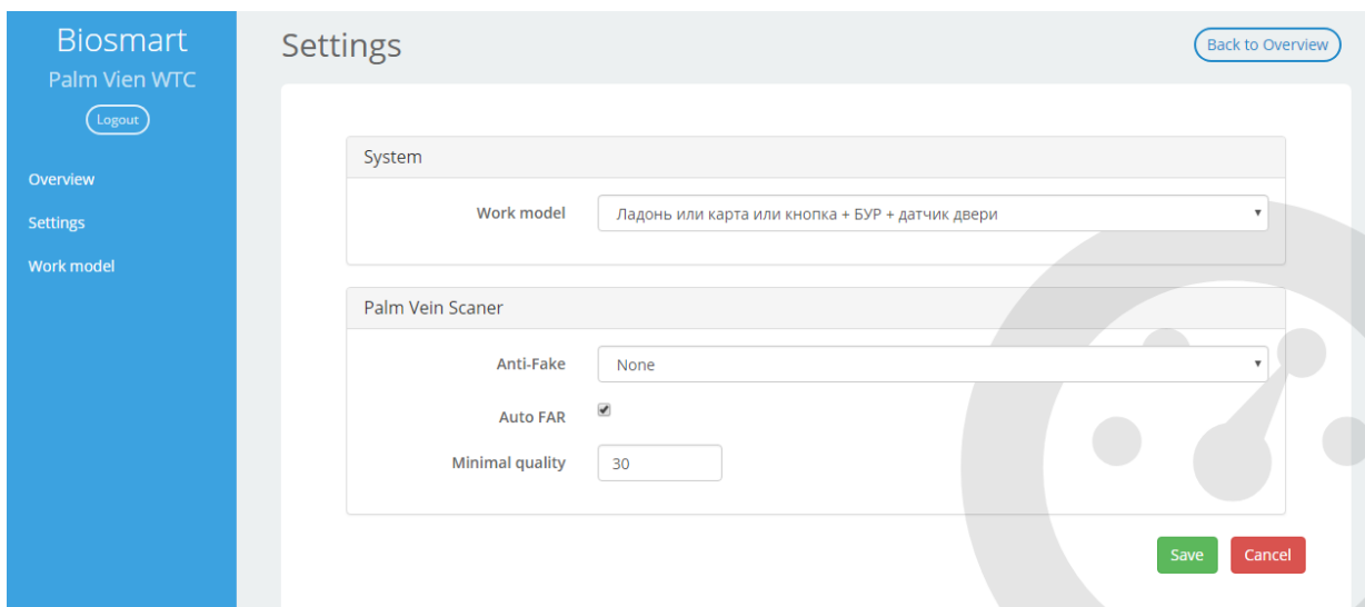
Рисунок 45. Раздел Settings
