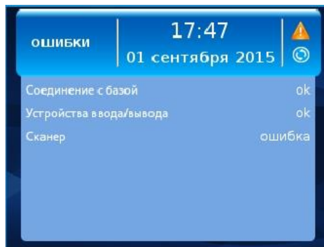
Рисунок 75. Ошибка сканера
