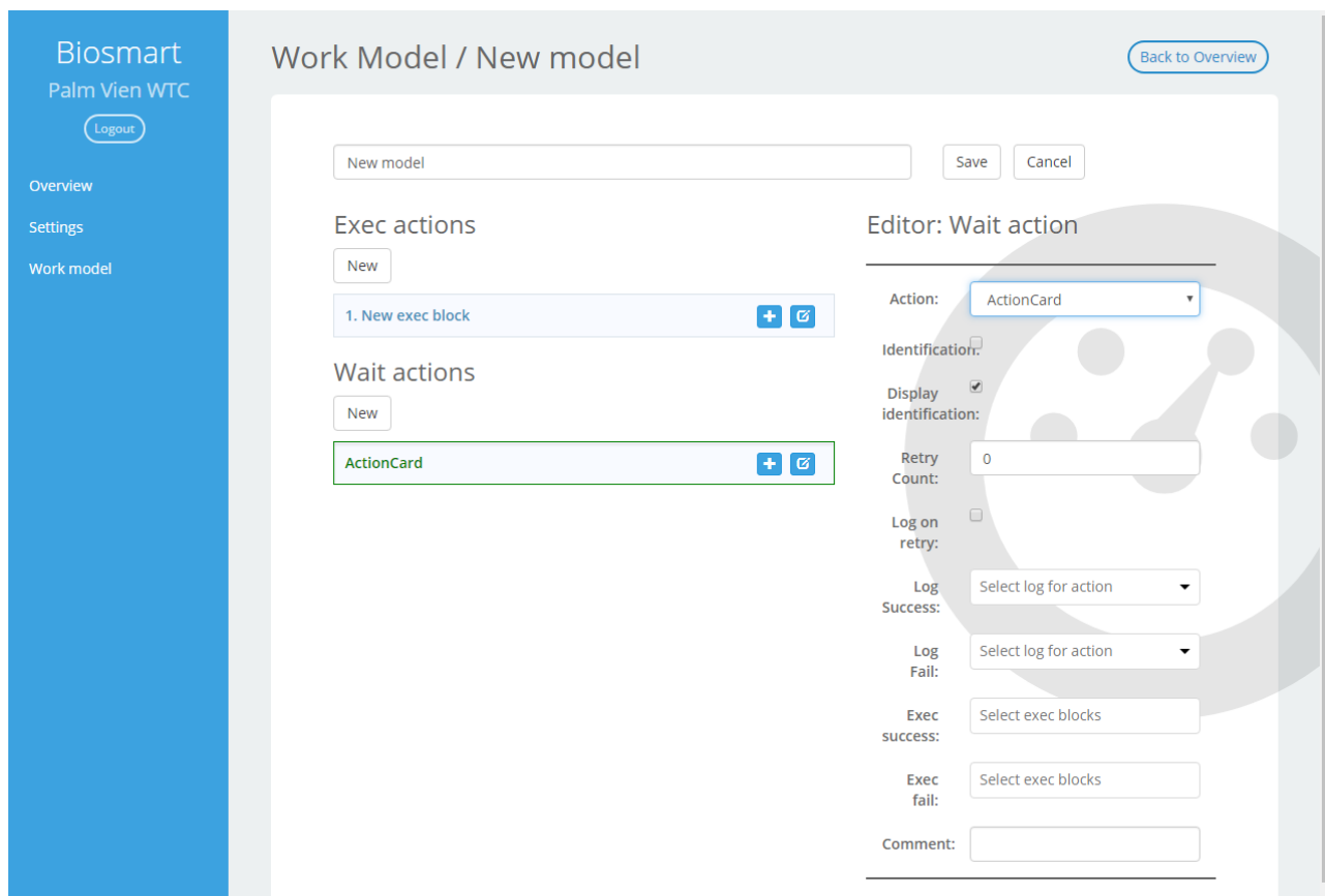
Рисунок 50. Блок событий
