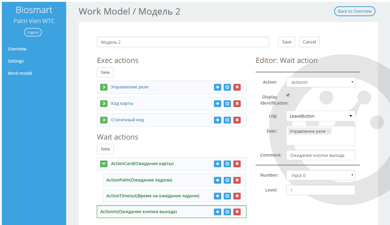
Рисунок 74. Создание сценария
