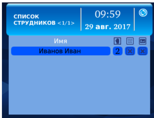
Рисунок 27. Список сотрудников
