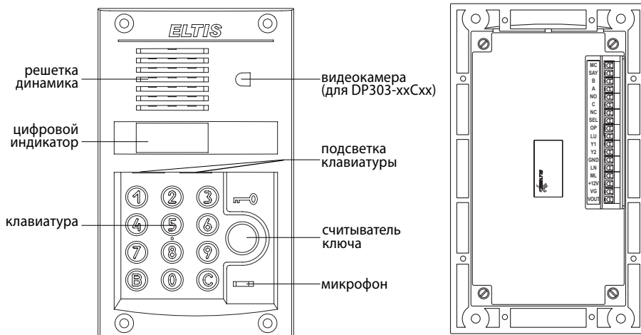
Рис.16 Внешний вид блоков вызова DP303-RD(C)24 и DP303-TD(C)22
