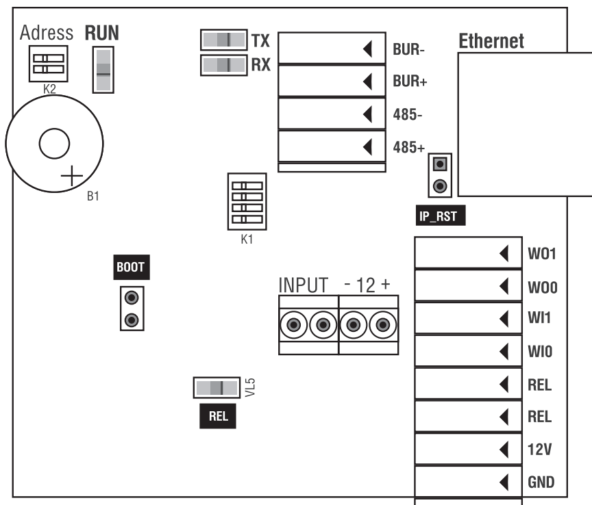
Рисунок 2. Внешний вид печатной платы клеммника
