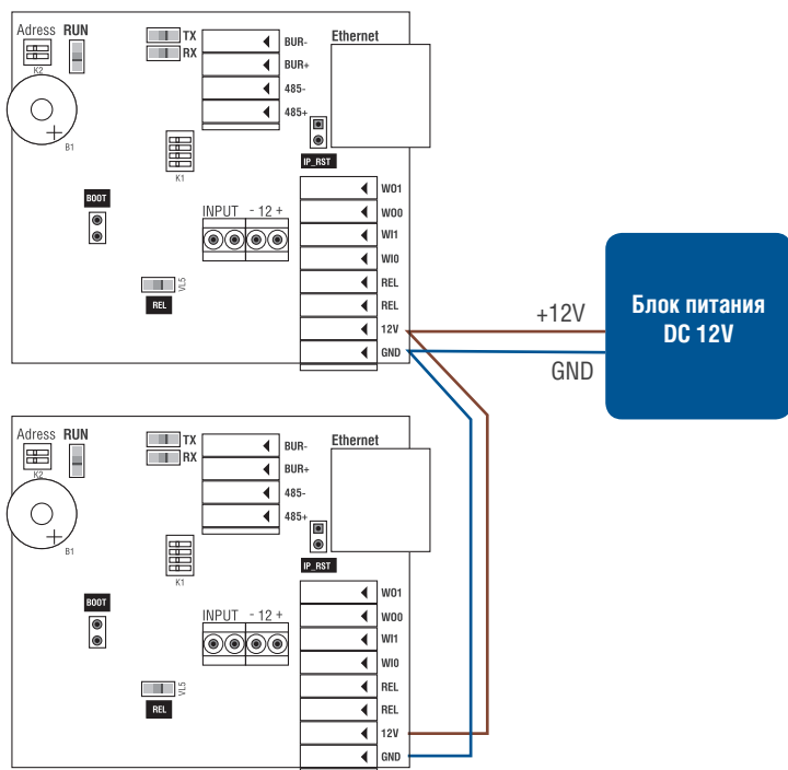
Рисунок 4. Схема подключения питания контроллера
