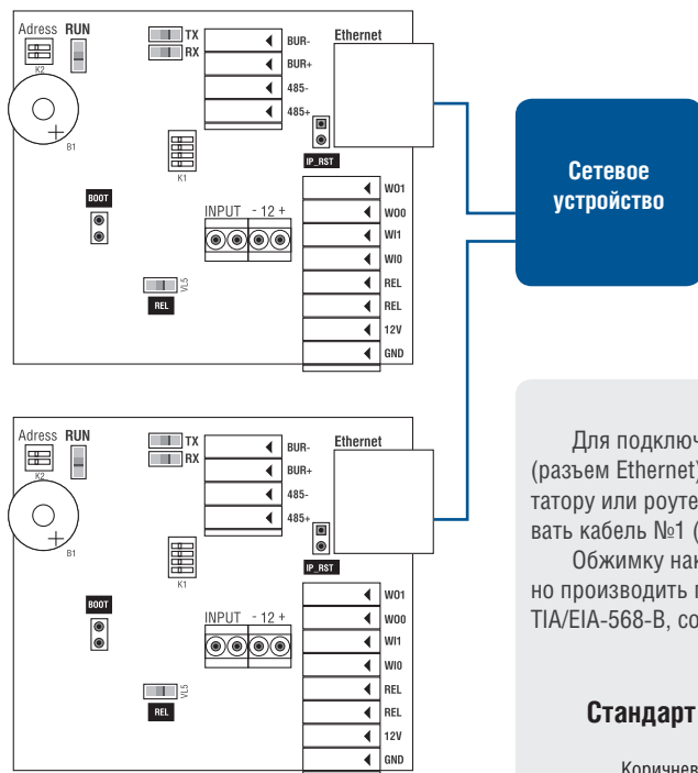
Рисунок 5. Схема подключения к сети Ethernet
