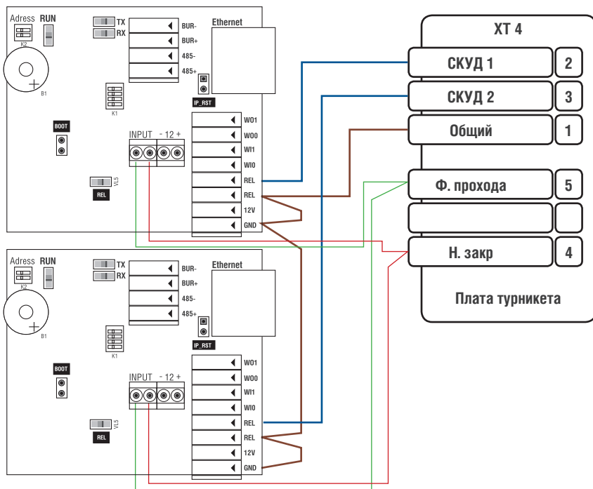
Рисунок 8. Схема подключения к турникету без использования БУР
