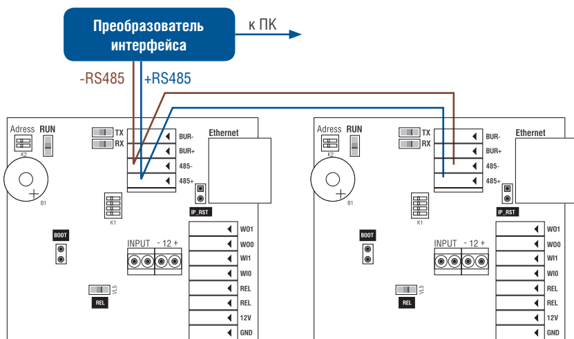
Рисунок 7. Схема подключения к преобразователю интерфейса.
