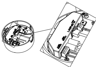
Рисунок 2-9 Подключение кабелей
