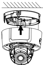
Рисунок 2-10 Закрепите корпус камеры
