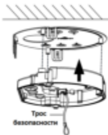
Рисунок 2-8 Установка распределительной коробки
