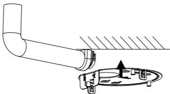
Рисунок 2-5 Установка кабельного канала
