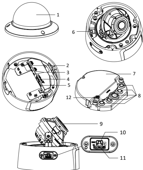
Рисунок 1-1 Обзор скоростной поворотной камеры
