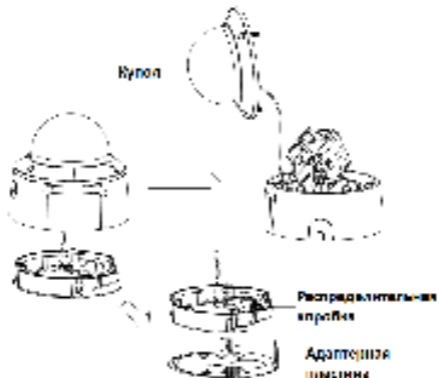
Рисунок 2-2 Разбор камеры
