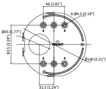
Рисунок 2-3 Адаптерная пластина
