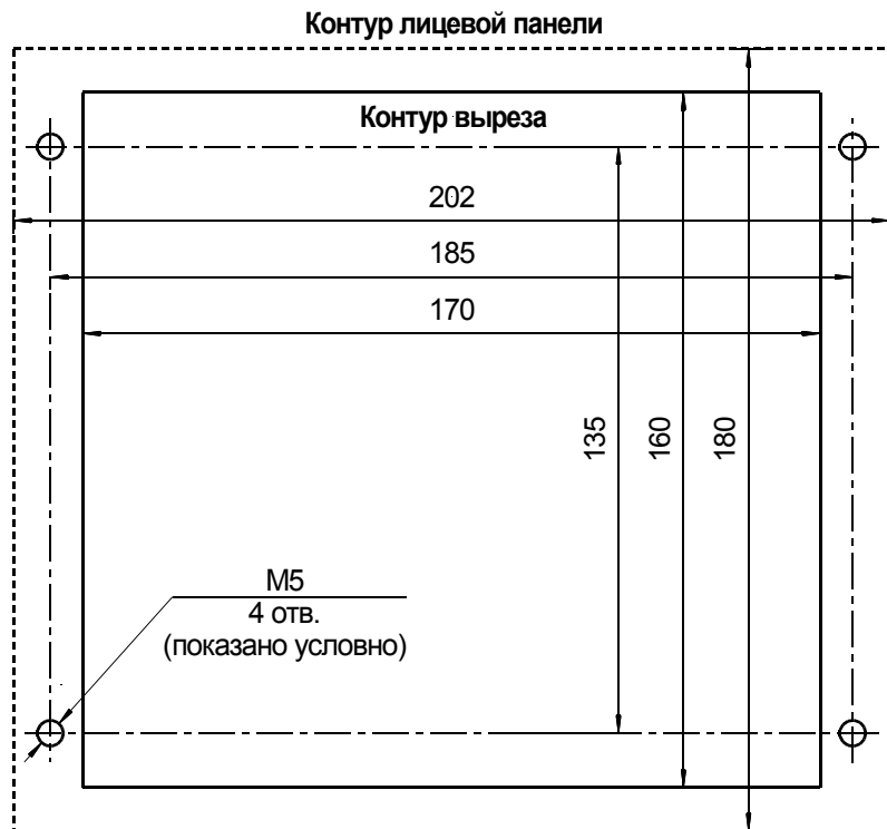
Рис. 1. Разметка под установку блока вызова.
